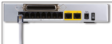
RJ-11-telefoonpoort
